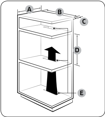
Mueble empotrado (mm)
