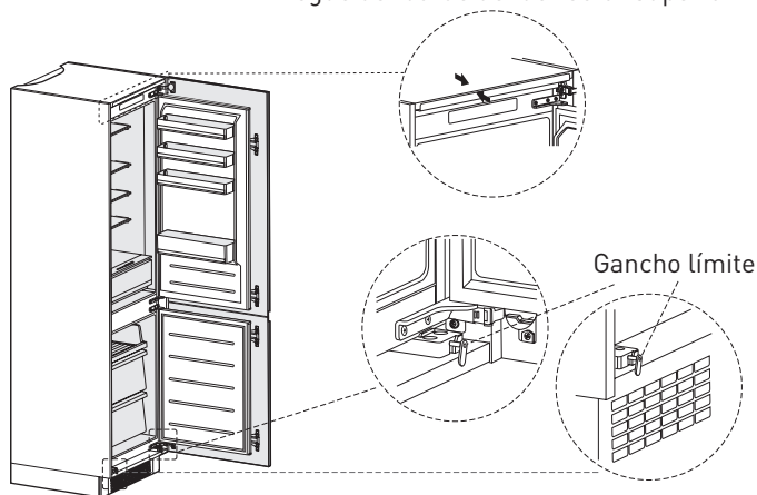
Pliegue del borde del deflector superior
